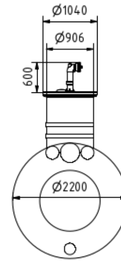
front view Ansicht von vorn
