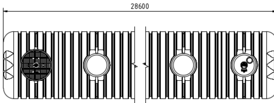
top view shortened Ansicht von oben verkürzt
