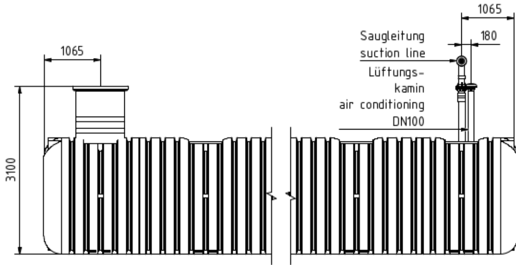
righthand view shortened Ansicht von rechts verkürzt
