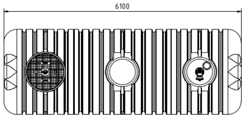
top view Ansicht von oben
