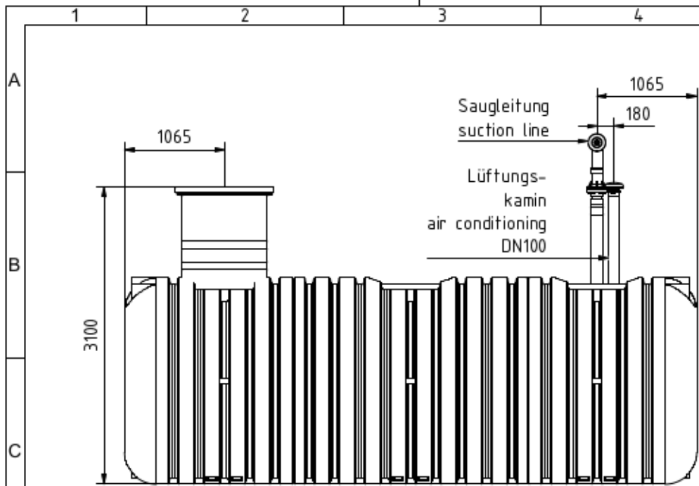
righthand view Ansicht von rechts
