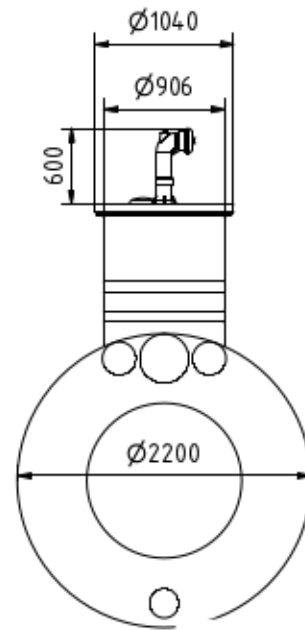
front view Ansicht von vorn
